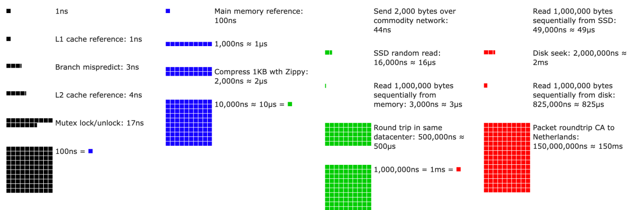
图12.4.1: 每个程序员都应该知道的延迟数字
