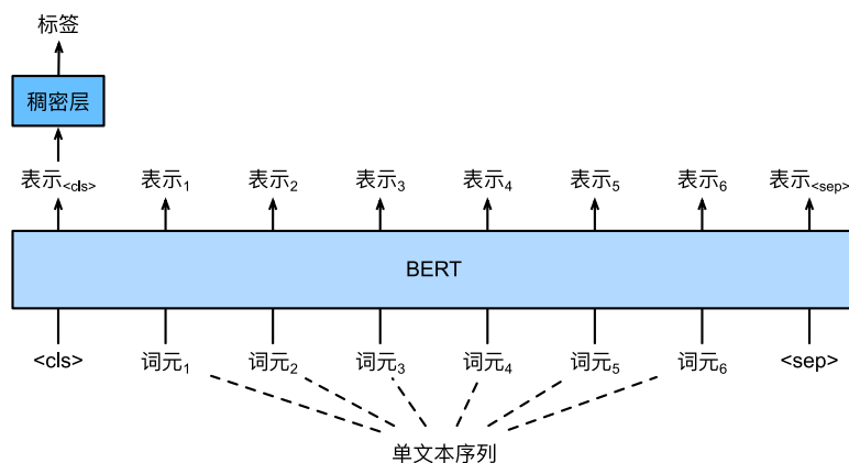
图15.6.1: 微调BERT用于单文本分类应用，如情感分析和测试语言可接受性（这里假设输入的单个文本有六个词元）
