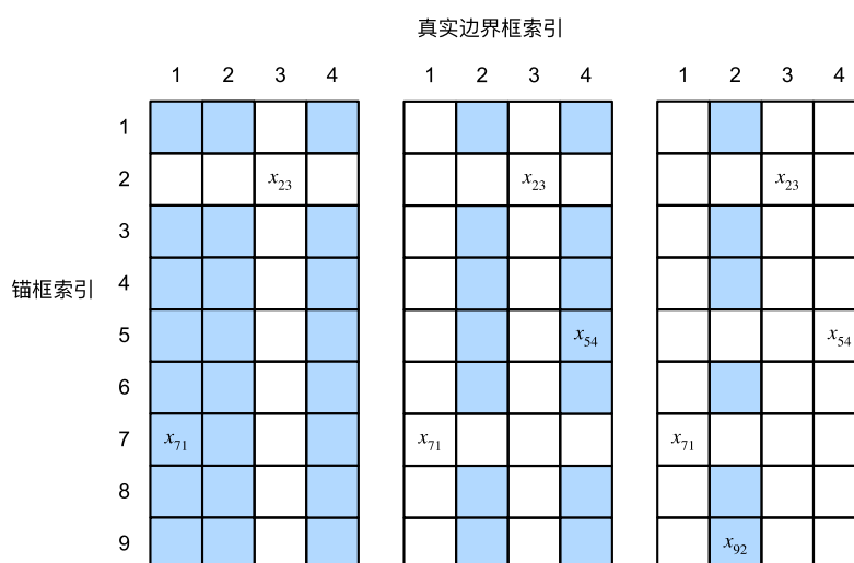
图13.4.2: 将真实边界框分配给锚框。
