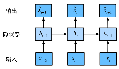
图8.1.2: 隐变量自回归模型
