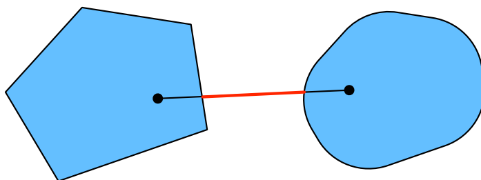
图11.2.3: 两个凸集的并集不一定是凸的。
