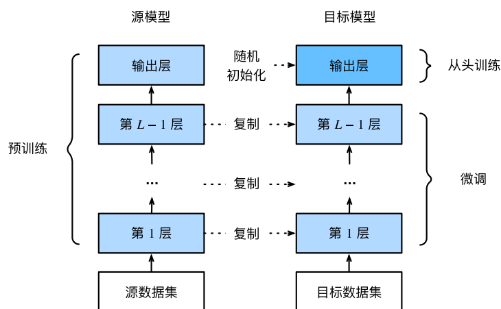
图13.2.1: 微调。
