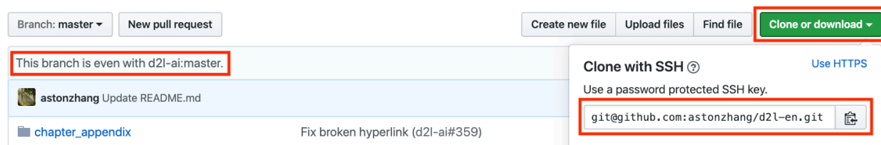
图16.5.5: 克隆存储库
