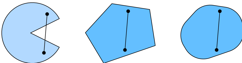
图11.2.1: 第一组是非凸的, 另外两组是凸的。
