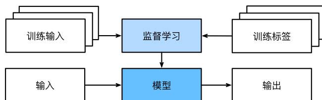
图1.3.1: 监督学习
