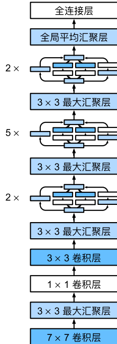
图7.4.2: GoogLeNet架构。
