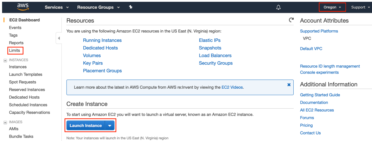
图16.3.2: EC2面板
