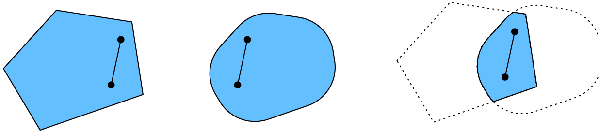
图11.2.2: 两个凸集交集是凸的。
