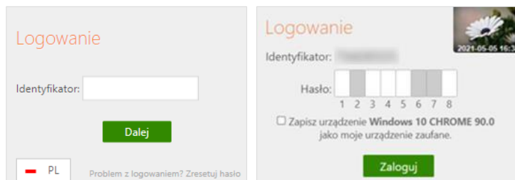
Rys.1 Okna „Logowanie”.
