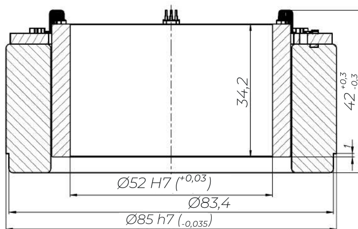
Схема электродвигателя
