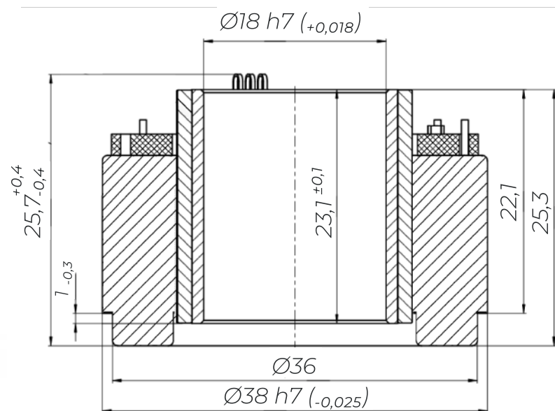
Схема электродвигателя
