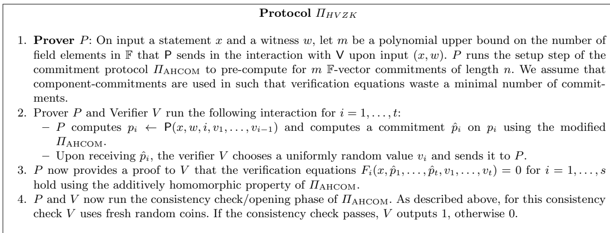
Fig. 15. Protocol \Pi_{\text{HVZK}}
