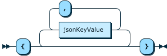
Figure 12.17 jsonDoc
