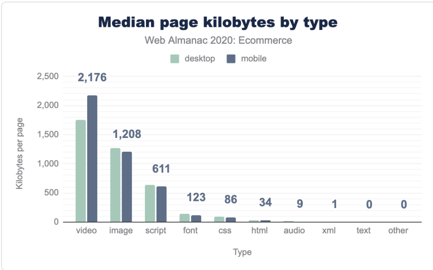
図16.10. タイプ別ページキロバイトの中央値
