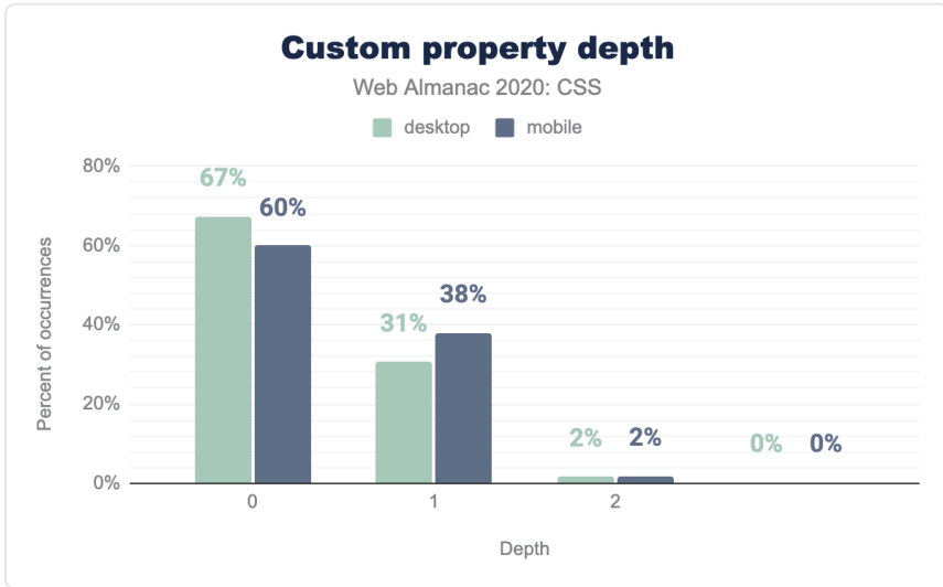
図1.49. カスタムプロパティの深さの分布を出現率で表したものの。
