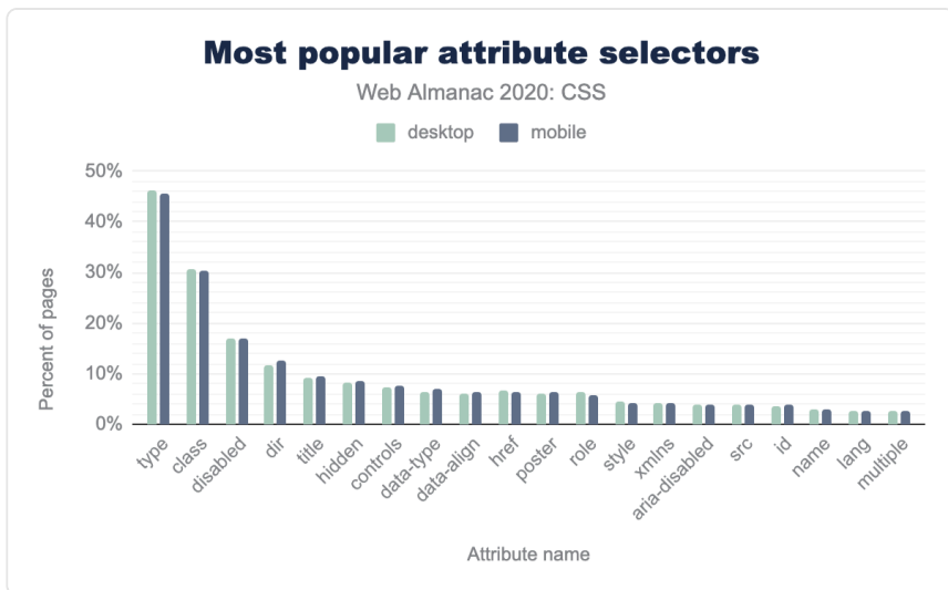
図1.11. ページの割合で最も人気のあるセレクター属性。
