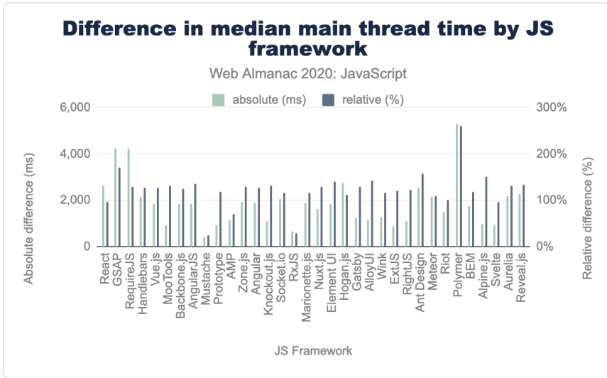
図2.27. デスクトップとモバイルの1ページあたりのメインスレッド時間の中央値の差 Ember.jsを除くJavaScriptフレームワーク別。
