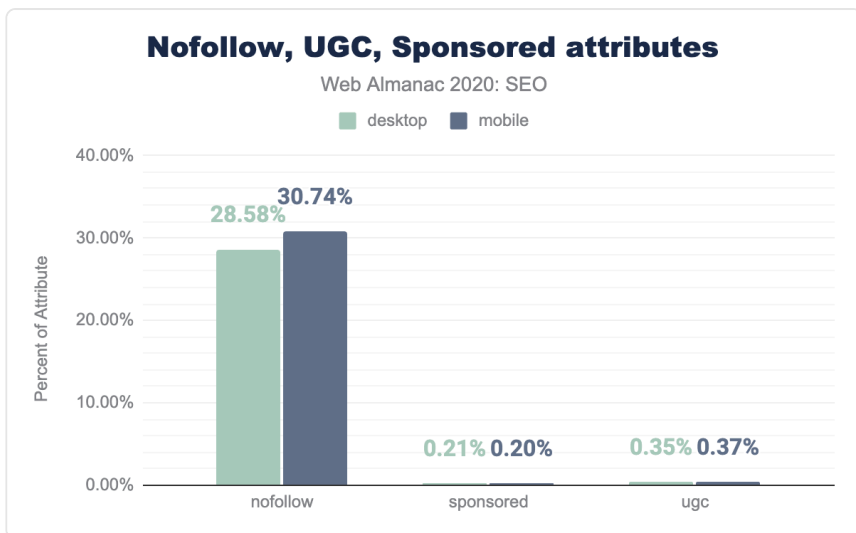
図7.24. rel=nofollow 、 rel=ugc 、 rel=sponsored の属性を持つページの割合です。
