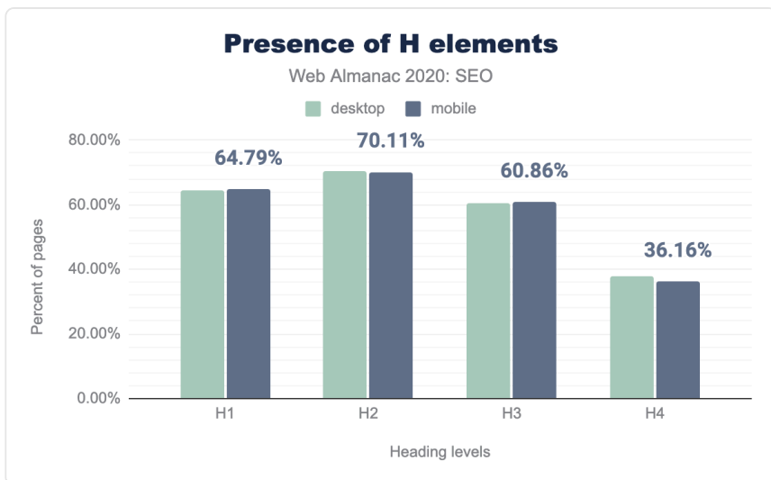
図7.8. 空の見出しを含む、見出しレベル1から4の使用。
