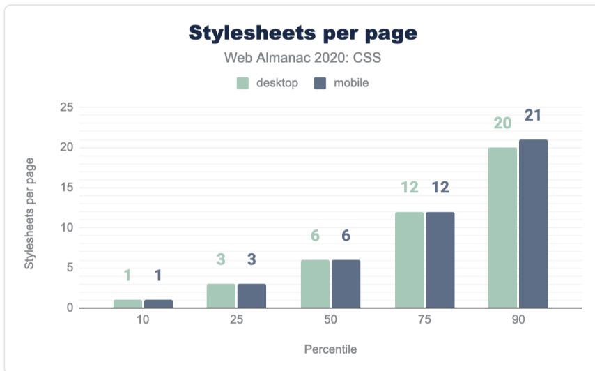
図1.3. 1ページあたりのスタイルシート数の分布。
