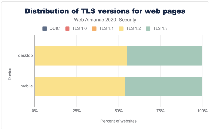
図11.4. サイトのTLSバージョンの使用状況
