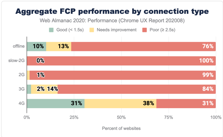
図9.16. 接続タイプ別に分割されたFCPのパフォーマンスを集計したものの。
