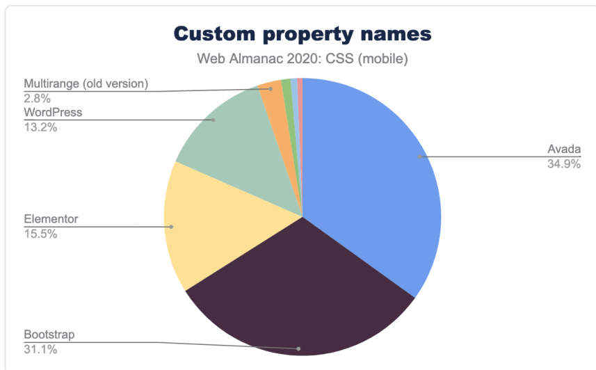
図1.46. ソフトウェアエンティティごとのカスタムプロパティ名の相対的な人気度を、モバイルページでの出現率として示しています。
