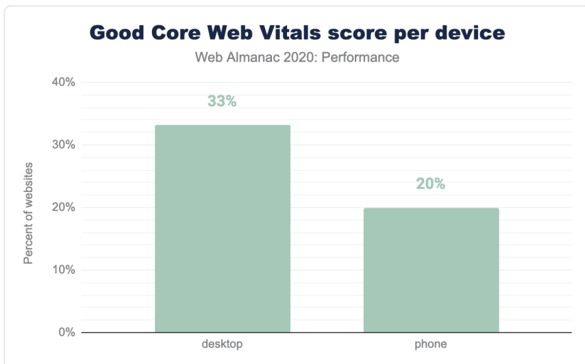
図7.27. デバイスごとのCore Web Vitals評価に合格したウェブサイトの割合。
