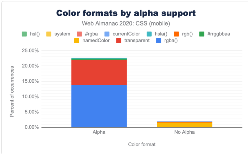
図1.26. カラーフォーマットの相対的な人気度をアルファサポート別にグループ化し、モバイルページでの出現率で示したもの（#rrggbb および #rgb を除く）。
