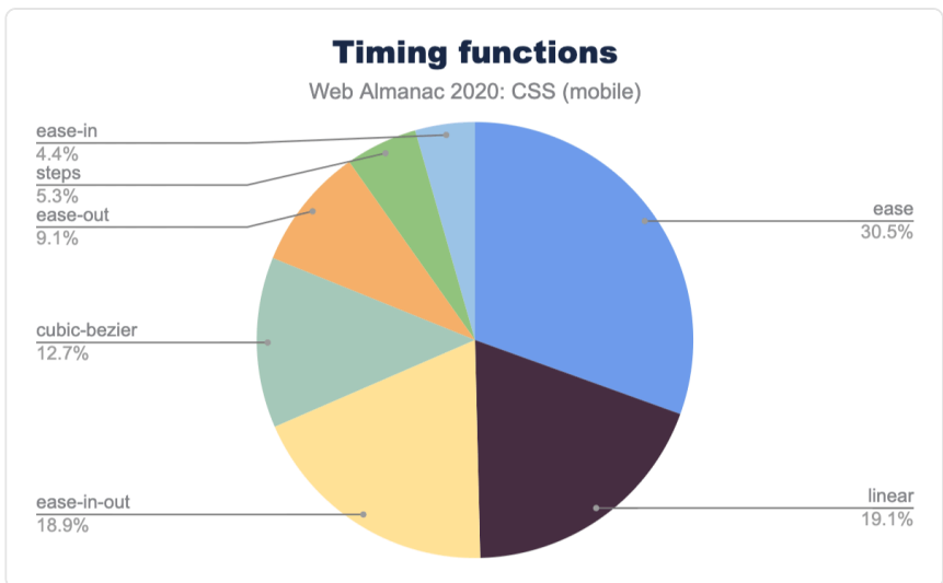
図1.40. タイミング機能の相対的な人気度は、モバイルページでの出現率として示されています。
