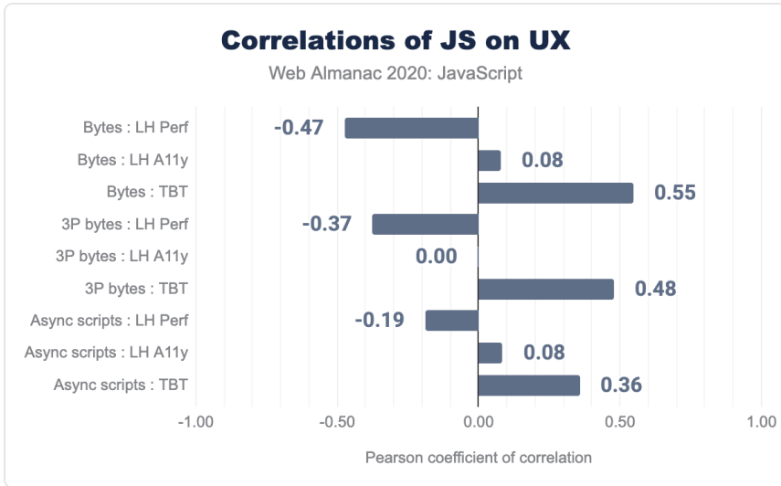
図2.29. ユーザー体験の様々な側面におけるJavaScriptの相関関係。
