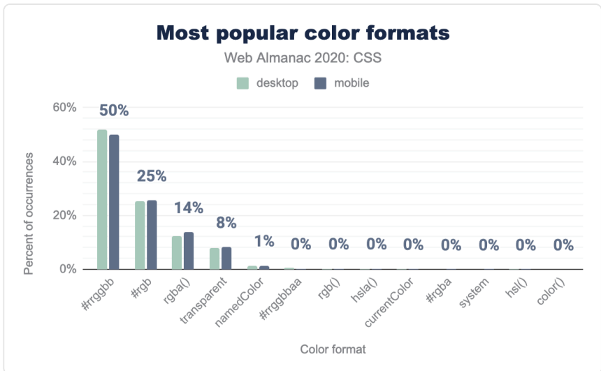
図1.25. カラーフォーマットの相対的な普及率。
