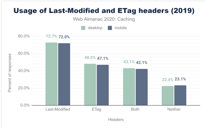
図20.8. 2019年には、 Last-Modified と ETag ヘッダーによる新鮮さの検証を採用。
