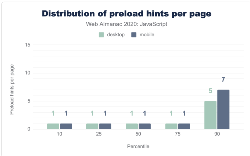
図2.15. 任意の preload ヒントを持つページあたりの preload ヒントの数の分布。
