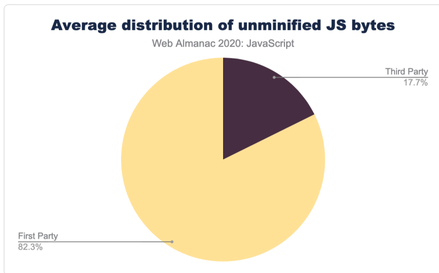
図2.17. ホスト別の最小化されていないJavaScriptのバイト数の平均分布。
