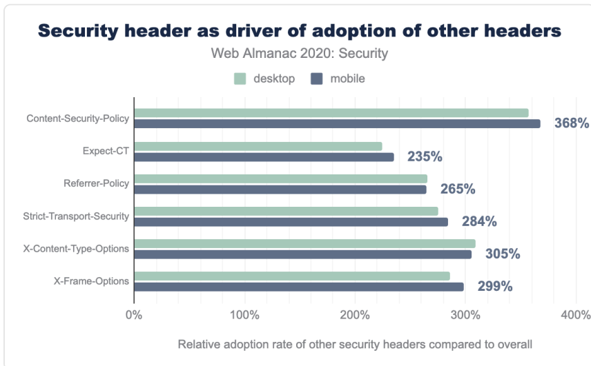
図11.28. 他のヘッダーを採用する際のドライバーとしてのセキュリティヘッダー
