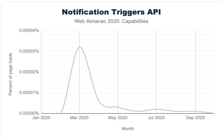
図13.5. Notification Triggers APIを使用したChromeでのページ読み込みの割合 (出典 通知トリガー 547 )
