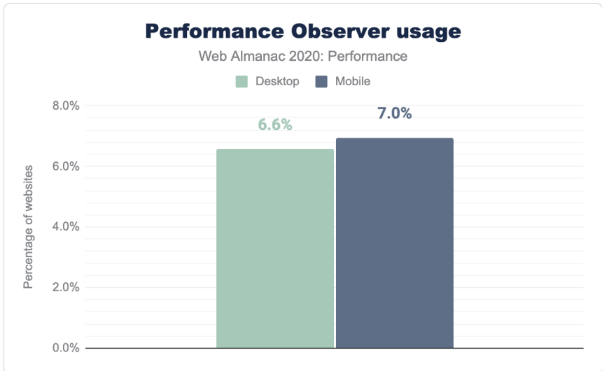
図9.20. パフォーマンス デバイスタイプ別のObserverの使用状況。
