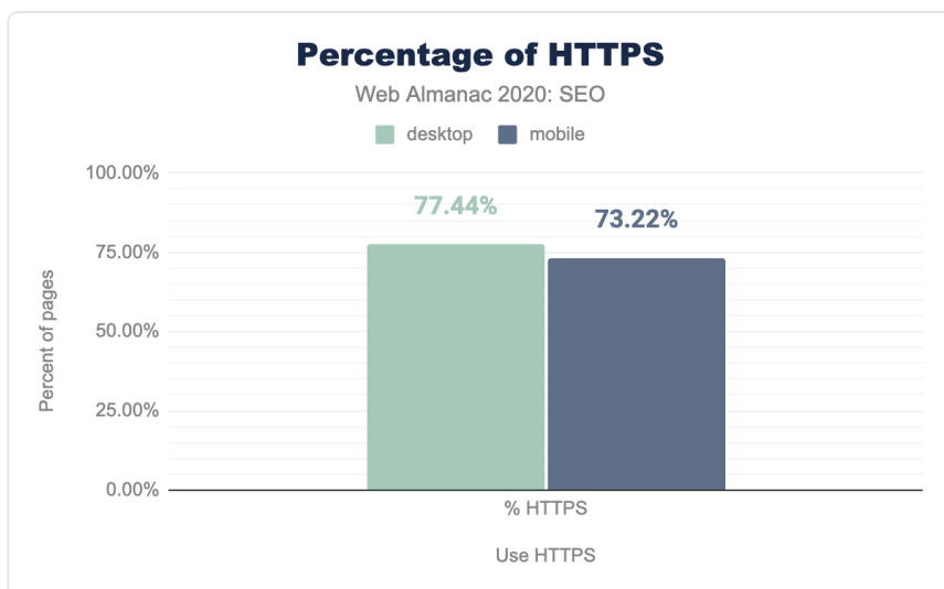
図7.33. HTTPSで提供されているページの割合。
