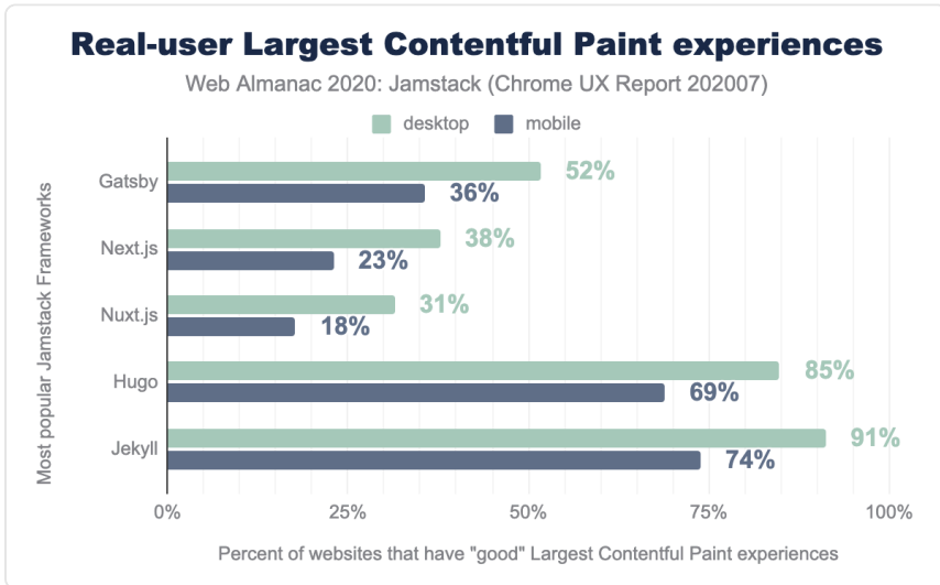
図17.9. リアルユーザー最大のコンテンツフルペイント体験談
