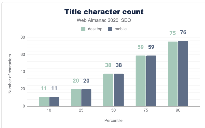
図7.12. ページタイトルごとの文字数の分布。
