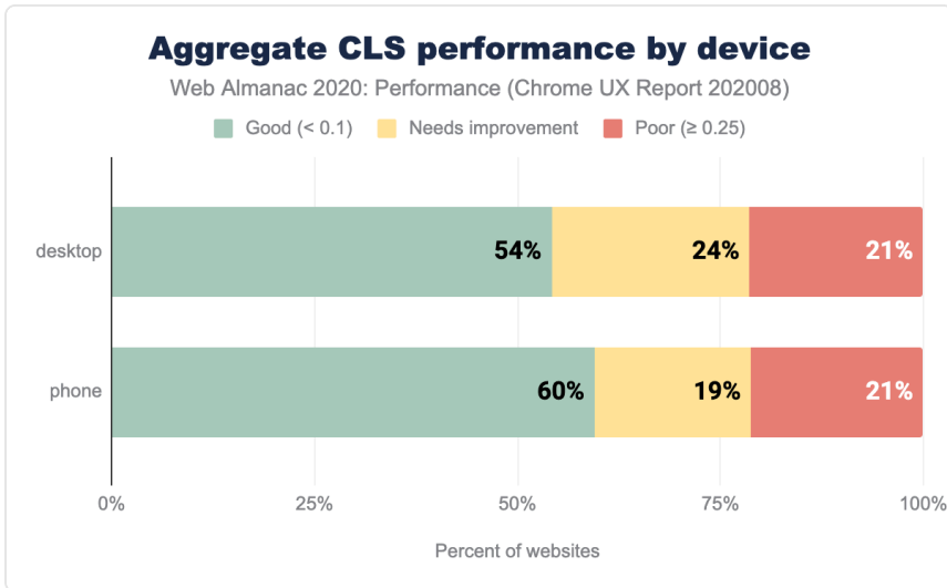
図9.6. デバイスタイプごとに分割されたCLSのパフォーマンスを集約。
