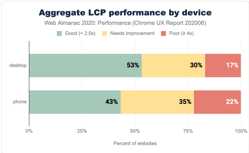
図9.3. デバイスタイプごとに分割されたLCPパフォーマンスの集計。
