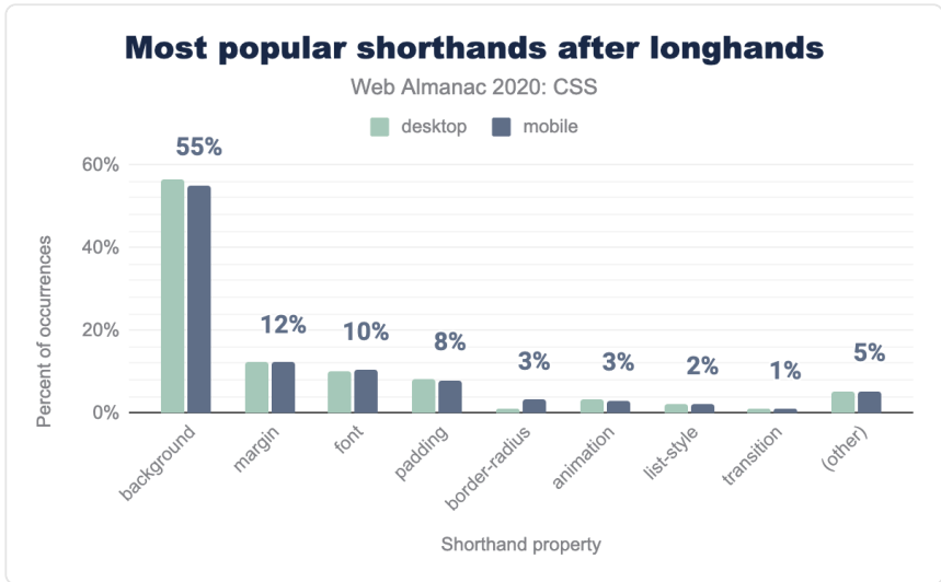
図1.70. 通常の記載の次に人気のある短縮形。
