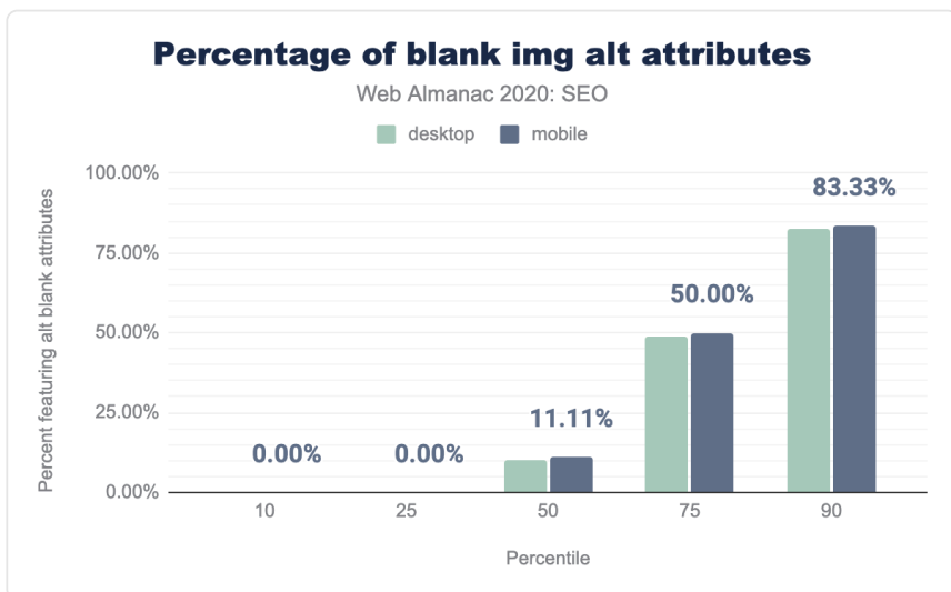
図7.18. 空白の alt 属性を持つイメージのページごとの割合の分布。
