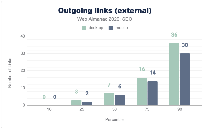
図7.21. ページごとの外部への発信リンク数の分布。
