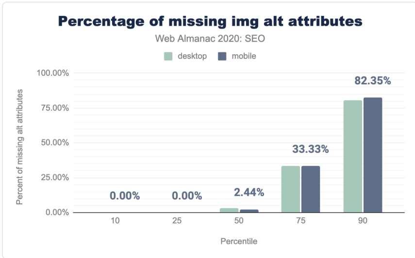
図7.16. イメージの alt 属性を欠く <img> 要素のページあたりの割合の分布。
