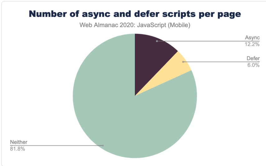
図2.13. モバイルページあたりの async および defer スクリプトの数の分布。
