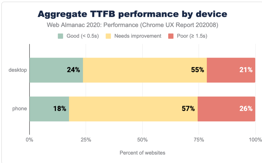
図9.17. デバイスタイプ別に分割されたTTFBのパフォーマンスを集計したものの。
