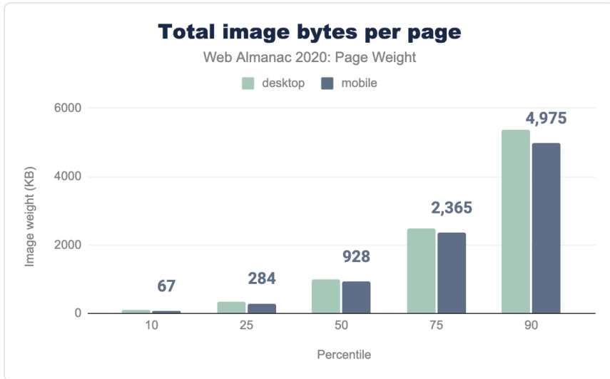
図18.6.1 ページあたりの画像レスポンスサイズの分布。
