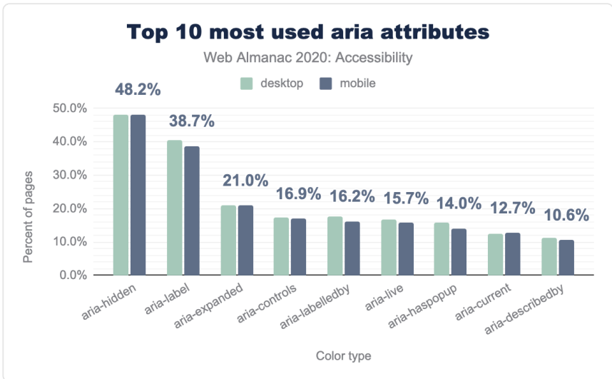
図8.17. 最もよく使われる aria 属性のトップ10。
