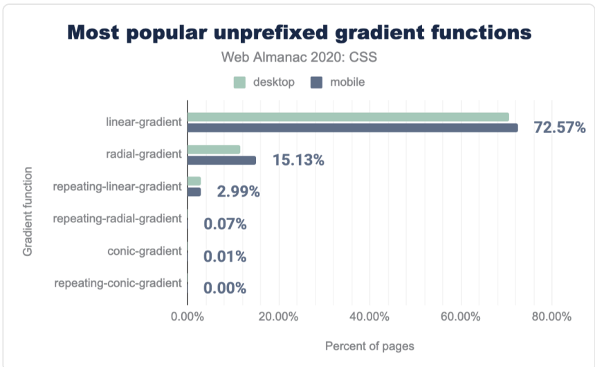
図1.32. 最も人気のあるグラデーションは、ベンダーの接頭辞を省略して、ページのパーセンテージとして機能します。
