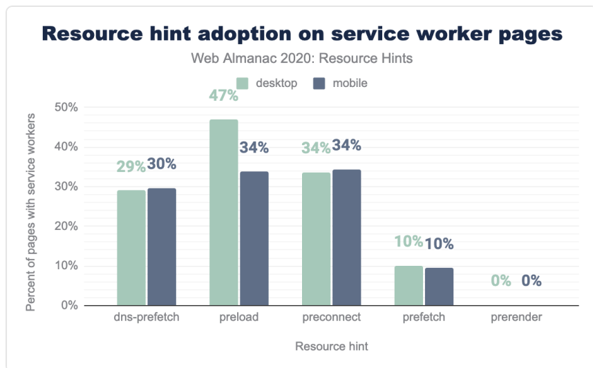
図21.10. サービスワーカーページでのリソースヒント採用。
