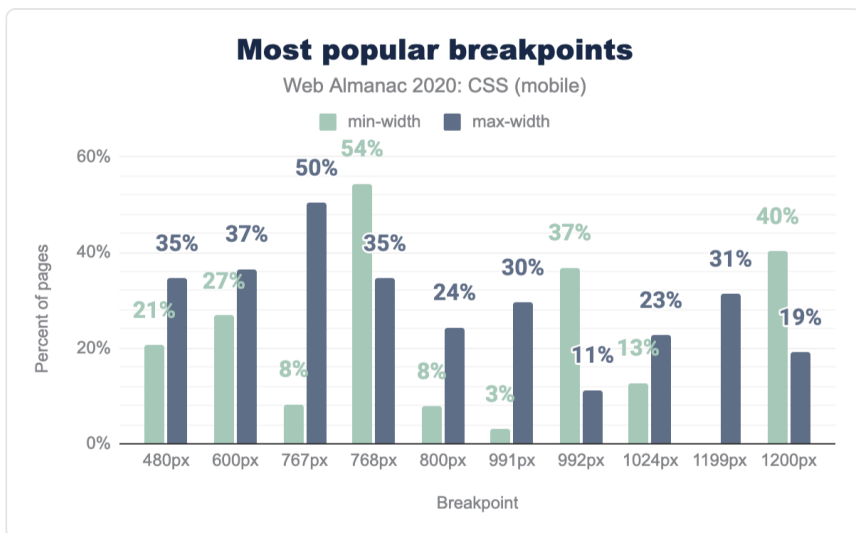
図1.44. モバイルページに占める割合として、 min-width と max-width による最も人気のあるブレイクポイントを示します。
