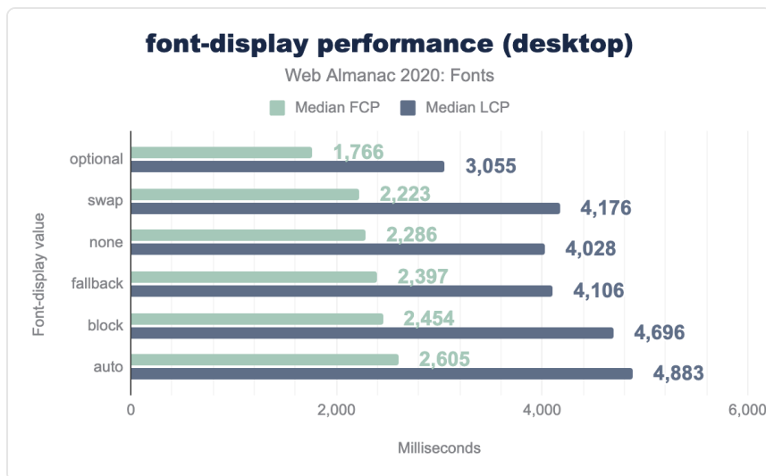
図4.10. デスクトップでの font-display のパフォーマンスを改善しました。
