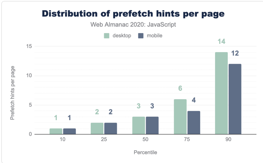
図2.14. 1ページあたりの prefetch ヒントの数の分布。
