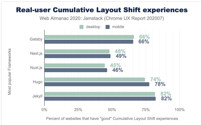
図17.11. リアルユーザーの累積レイアウト変更の体験
