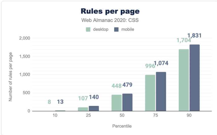
図1.4.1 ページあたりのスタイルルールの総数の分布。
