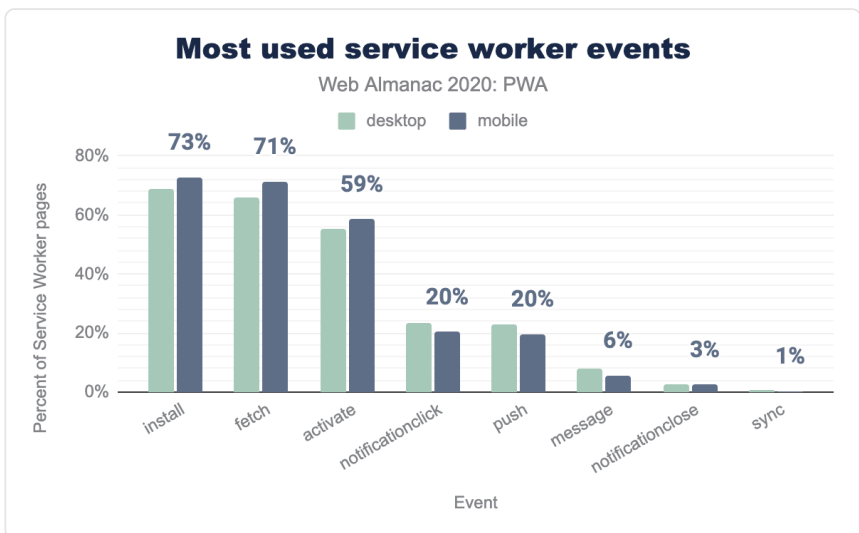
図14.3. もっとも利用されるサービスワーカーのイベント
