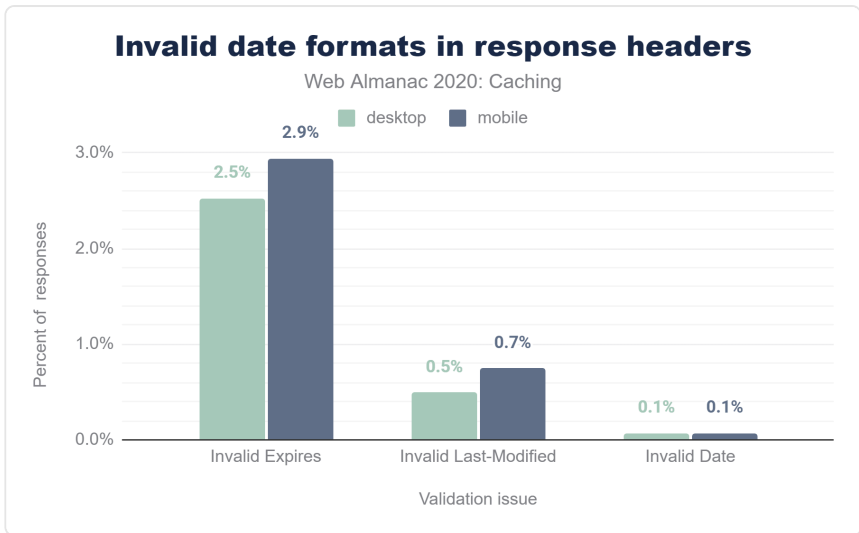
図20.10. レスポンスヘッダーの日付フォーマットが無効です。
