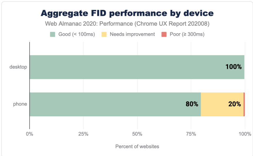
図9.9. デバイスタイプ別に分割されたFIDのパフォーマンスを集約したものの。
