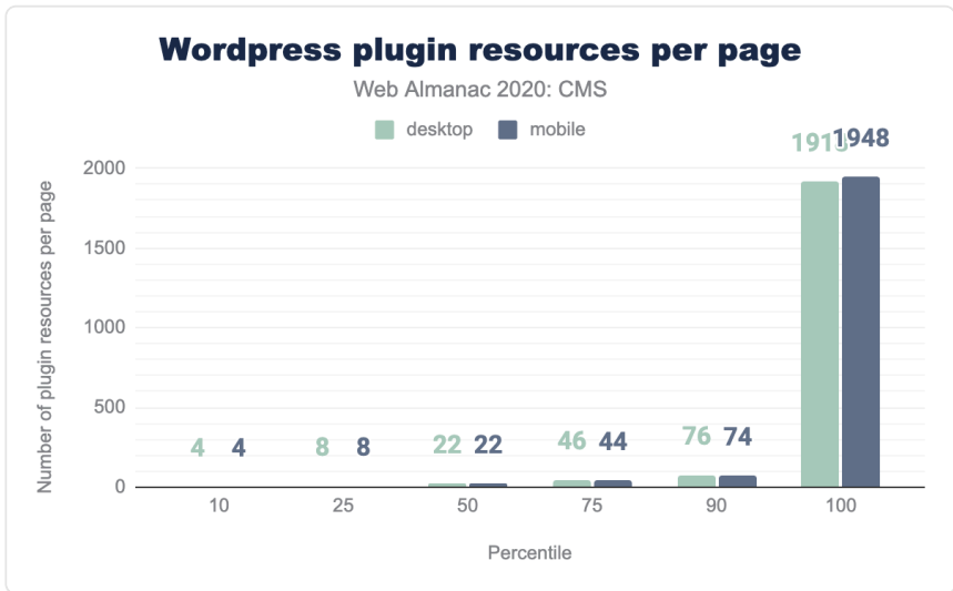
図15.7. ページごとのWordPressプラグインのリソース。
