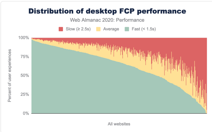
図9.12. デスクトップでのFCPパフォーマンスが「速い」「普通」「遅い」と判定されたウェブサイトの分布。
