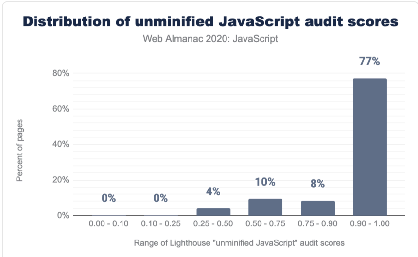
図2.16. 未定義のJavaScript Lighthouseの監査スコアをモバイルページごとに配布していません。
