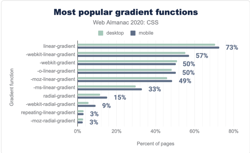
図1.31. ページのパーセンテージとして最も人気のあるグラデーション機能です。
