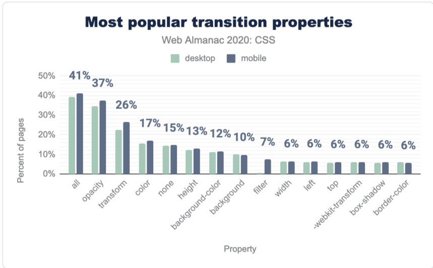
図1.38. ページの割合としてトランジションプロパティを採用しています。
