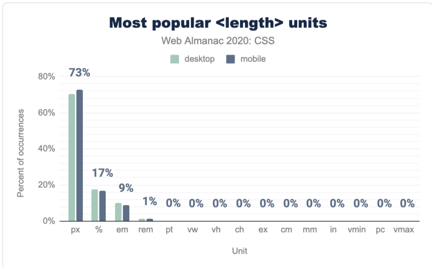
図1.16. 最も人気のある <length> の単位を出現率で表したものです。
