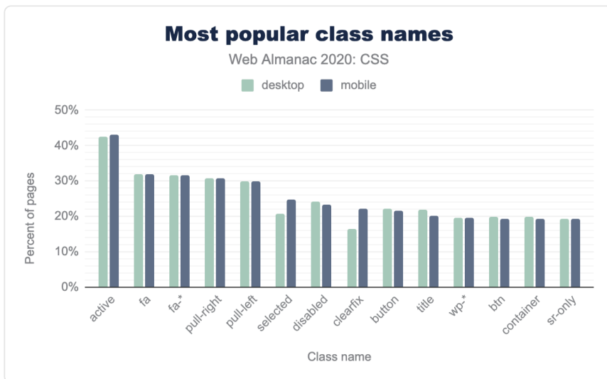
図1.5. ページ数の割合で最も人気のあるクラス名です。
