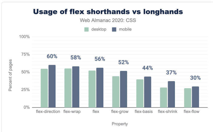
図1.67. flexの短縮形とその通常の記載の使い方比較
