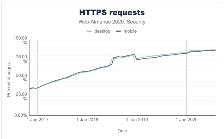
図11.2. HTTPSを使用したリクエストの割合 (出典。HTTP Archive 430 )
