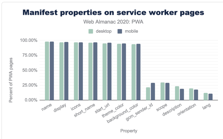
図14.5. サービスワーカーページのマニフェストプロパティ
