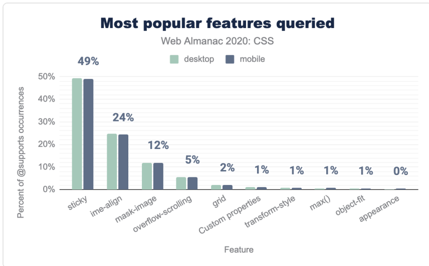
図1.61. サポート機能の相対的な人気度を、出現率として問い合わせました。
