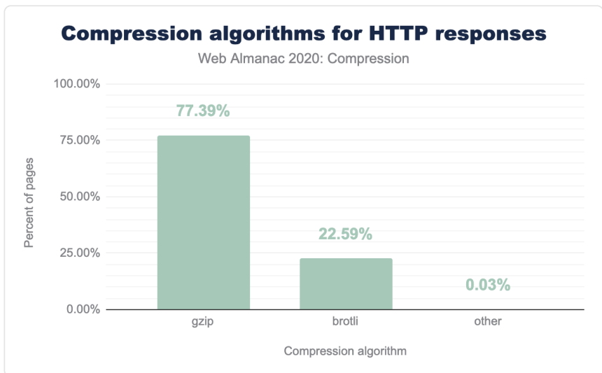
図19.5. HTTPレスポンスの圧縮アルゴリズム。
