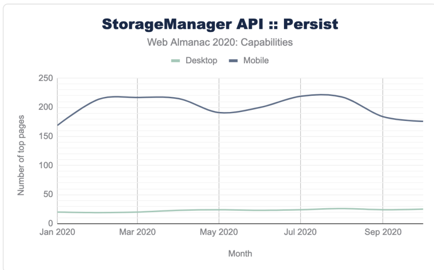
図13.3. StorageManager APIのpersistメソッドの使用ページ数。
