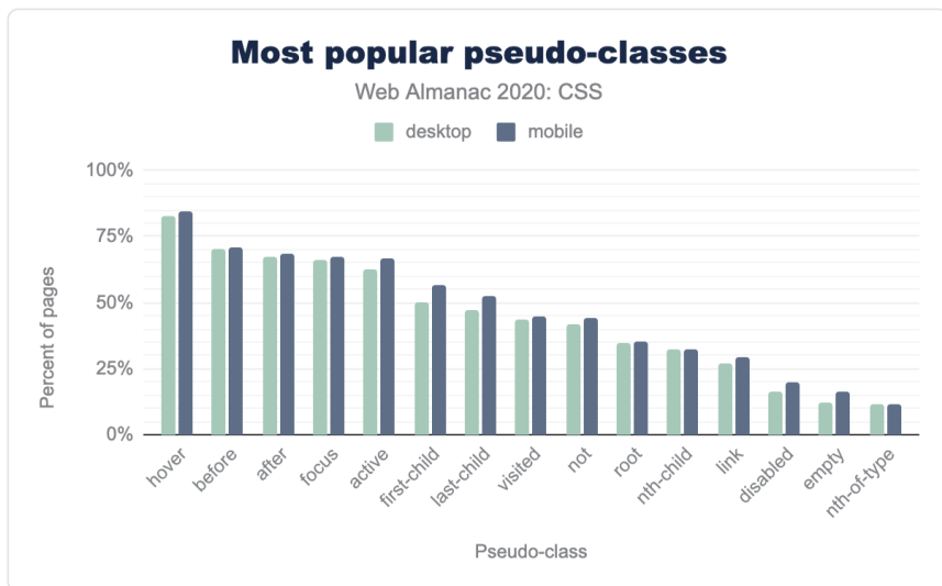
図1.13. ページ数に占める割合としては、最も人気のある疑似クラス。
