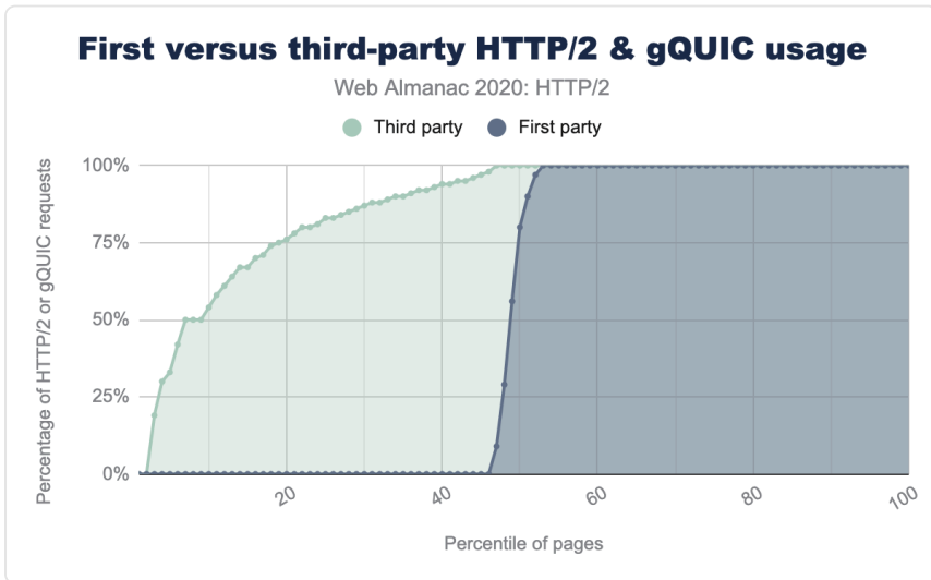
図22.7. 1ページあたりのサードパーティとファーストパーティのHTTP/2リクエストの割合の分布。
