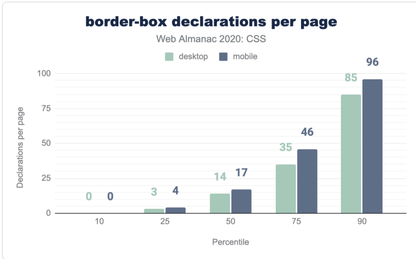
図1.37. 1ページあたりの border-box 宣言の数の分布。
