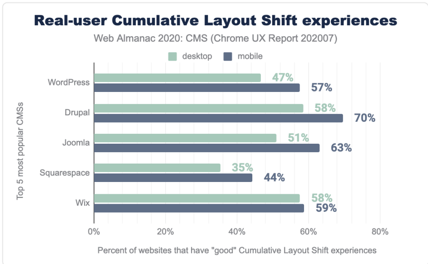
図15.10. 実際のユーザーによる累積レイアウト変更の体験。
