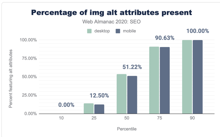
図7.17. ページごとの alt 属性を持つ画像の割合の分布。
