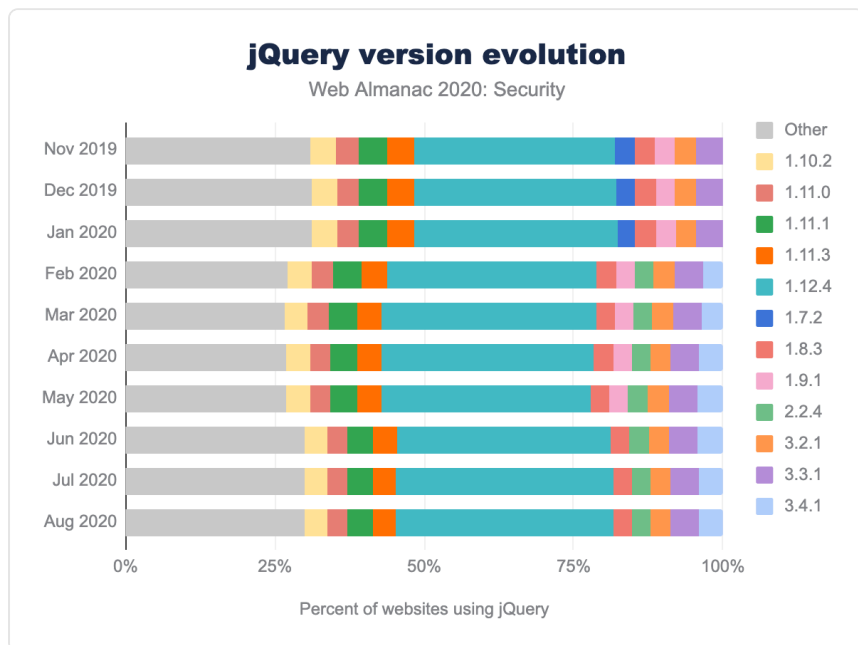
図11.31. jQueryのバージョンアップ。
