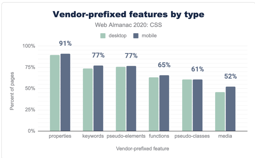
図1.53. タイプ別で最も人気のあるベンダープリフィックス機能をページ数に占める割合で表示しています。
