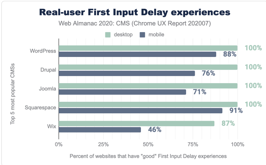
図15.9. 実際のユーザーによる初回入力遅延の体験
