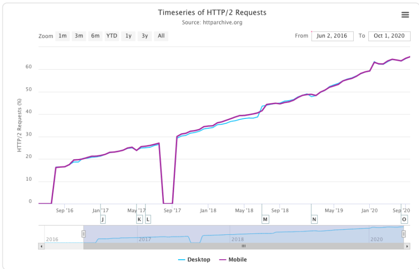
図22.1. リクエスト別のHTTP/2の使用状況。(提供元: HTTP Archive 755 )
