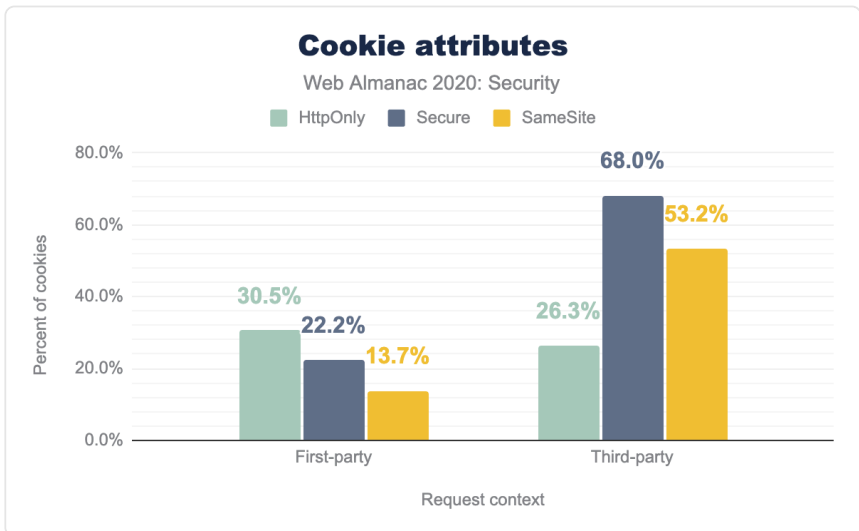
図11.11. Cookie属性。
