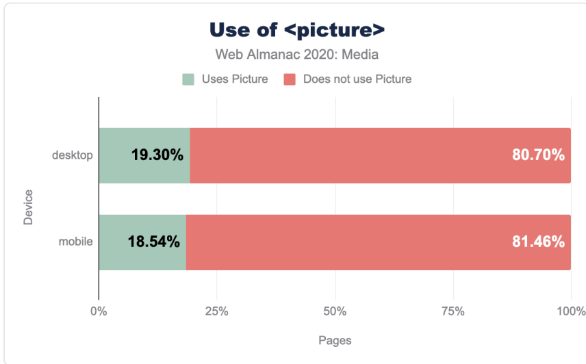
図5.4. <picture> の使用。
