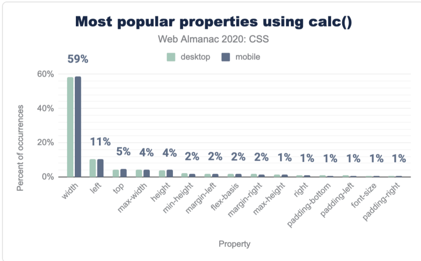
図1.20. calc() を使用するプロパティの相対的な人気度を、出現率の割合で示します。
