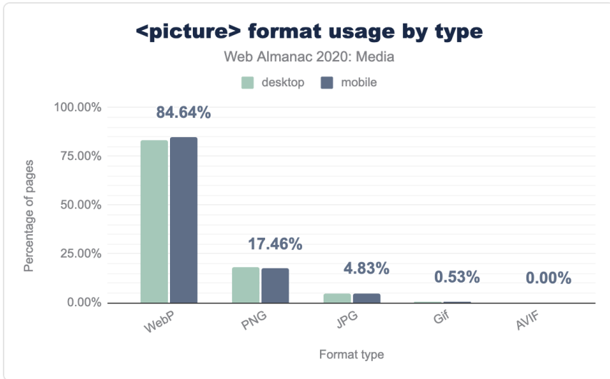
図5.6. タイプ別の写真フォーマットの使用状況
