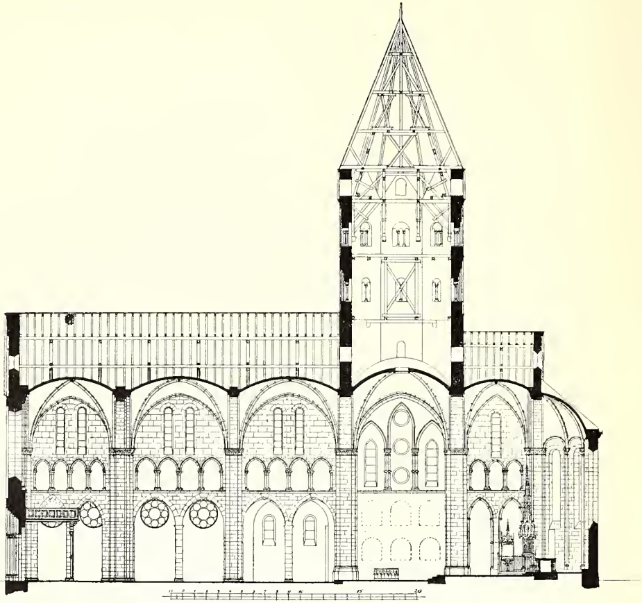
Fig. 37 Gerresheim. Längsschnitt der Stiftskirche.
