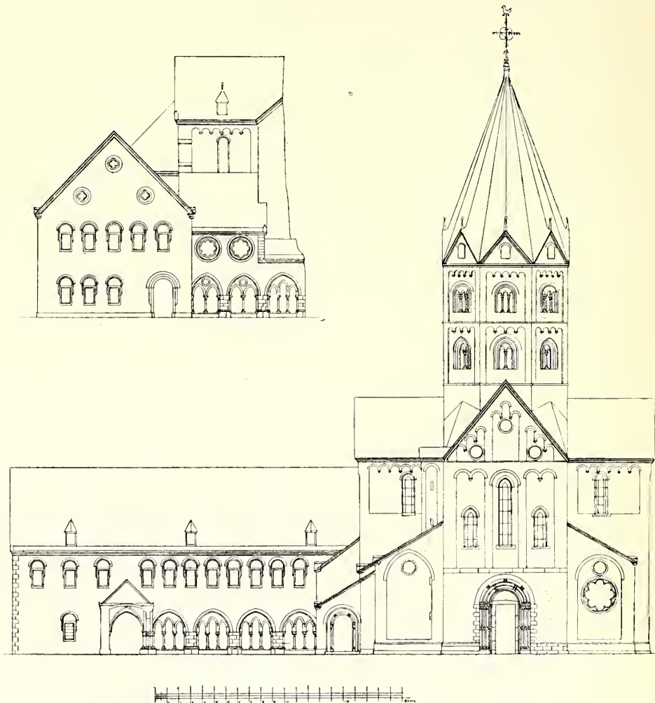
Fig. 35. Gerresheim. Westansicht der Stiftskirche, West- und Nordansicht des Kapitelhauses.
