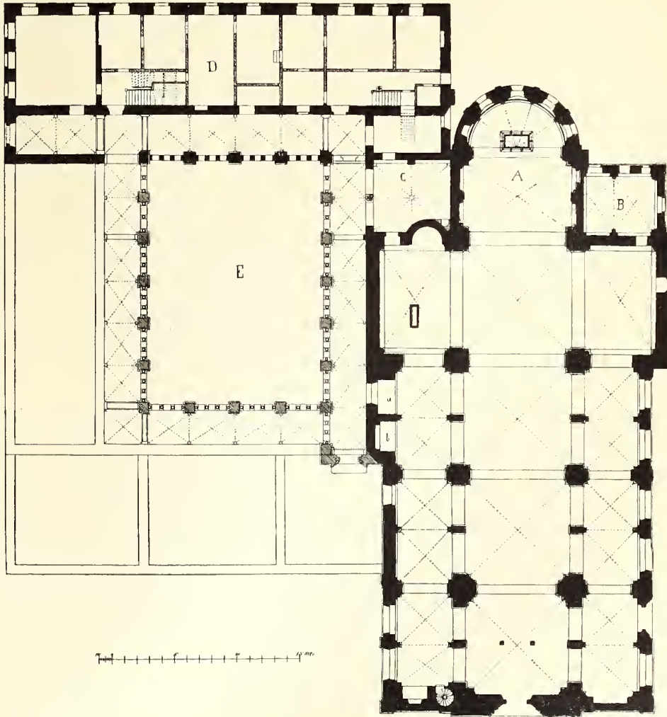
Fig. 34. Gerresheim. Grundriss der Stiftskirche mit Kapitelshaus und Kreuzgang.
