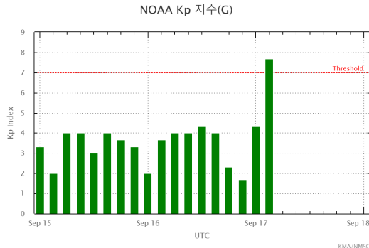
지구자기장 교란지수
