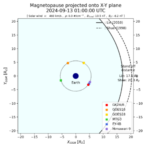
지구자기권계면의 위치
